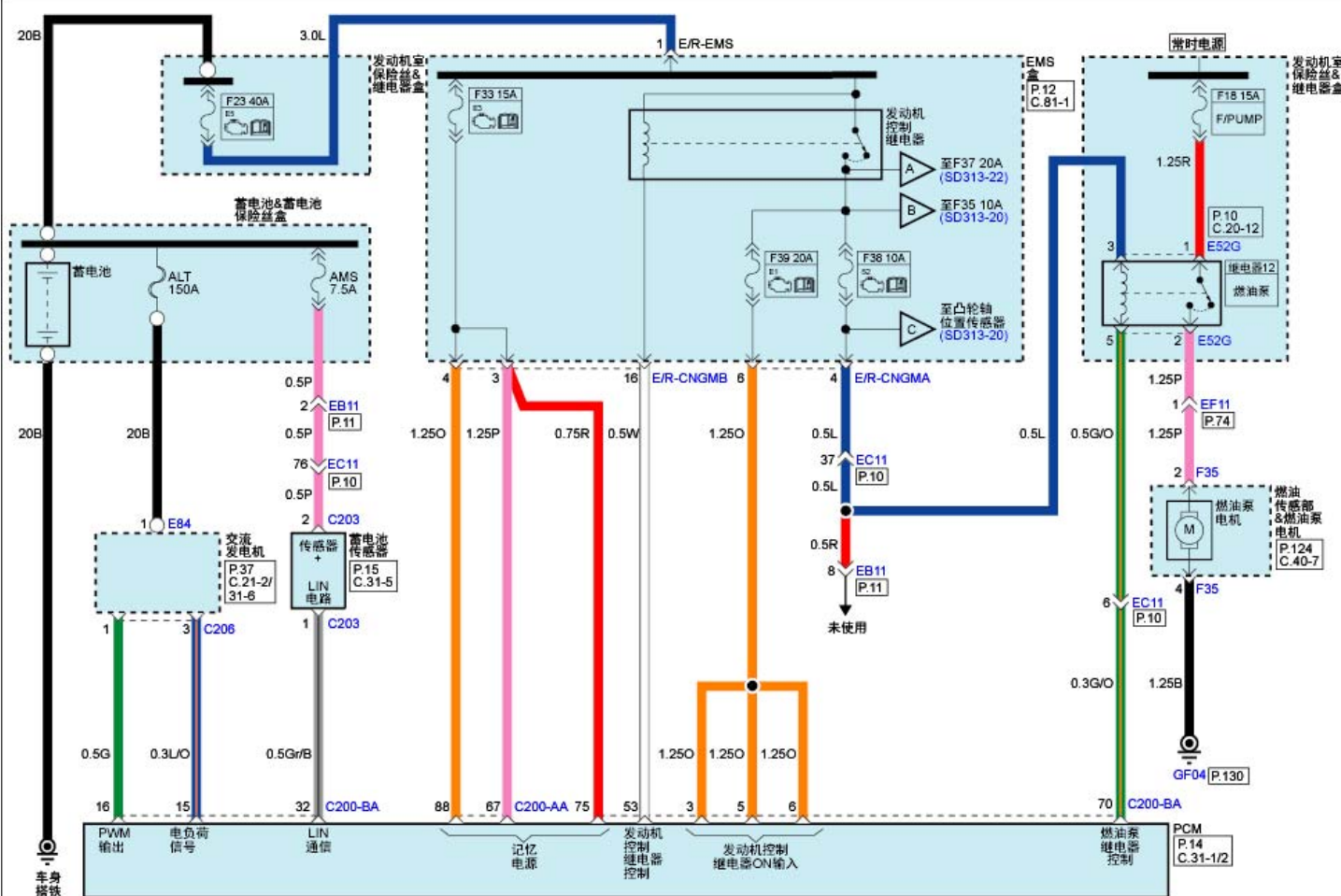
发动机控制系统(G4NA: NU 2.0L MPI A/T)(3)
